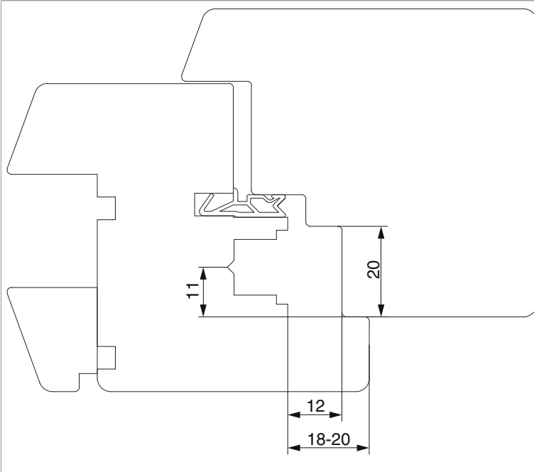
A12 battuta liscia PB20 scost.11 - 1 anta
