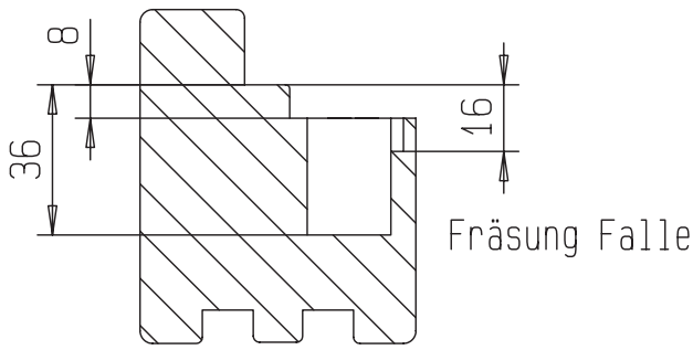
U-Schiene
