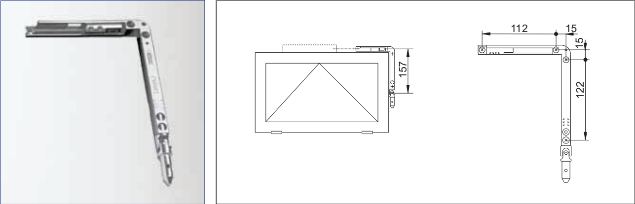
Finestre rettangolari con GEZE Fz 90
