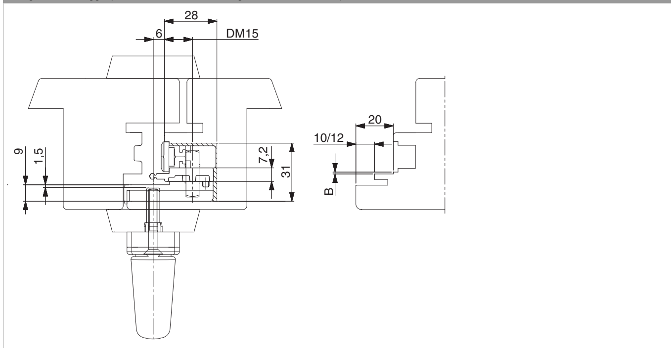
Disegno di montaggio profilo A12/AB20/sc. 9 con guarnizione in battuta piccola, distanza cava ferramenta 1 mm
