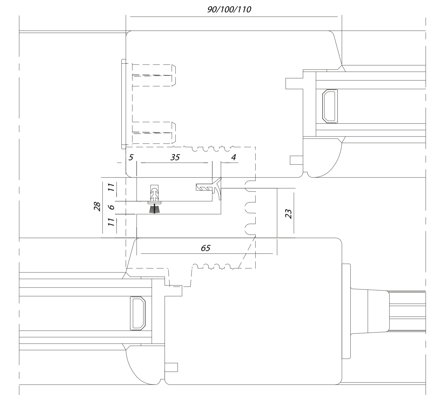
SOLUZIONE NODO CENTRALE CON LISTELLI IN LEGNO CLIMATECH EASY 68mm
