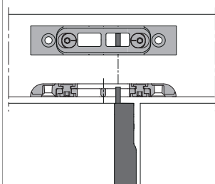
Porta a 2 ante con 1 catenaccio
