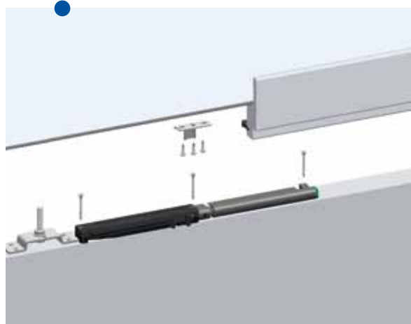
Particolare dell'accessorio Rallenty Soft installato sul pannello porta
