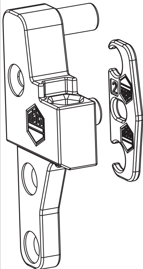
Montaggio spessore del sistema di supporto
