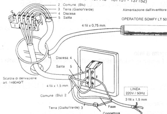
SCHEMA APPLICATIVO
