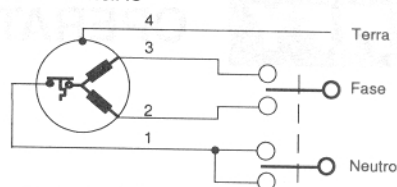
SCHEMA APPLICATIVO
