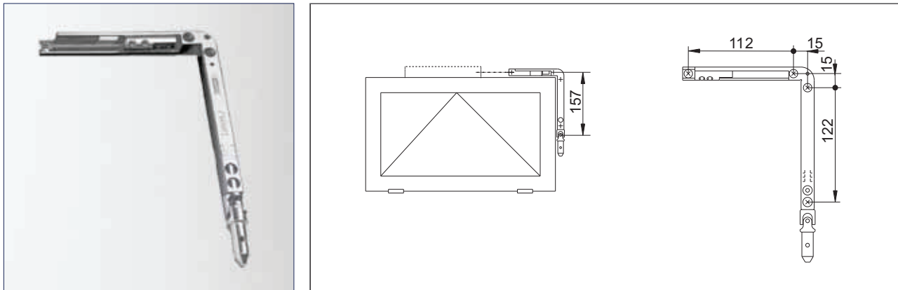
Finestre rettangolari con GEZE Fz 90
