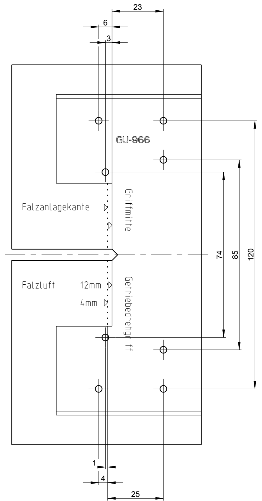
1 x 9-31955-00-0 Bohrschablone für Getriebedrehgriff
