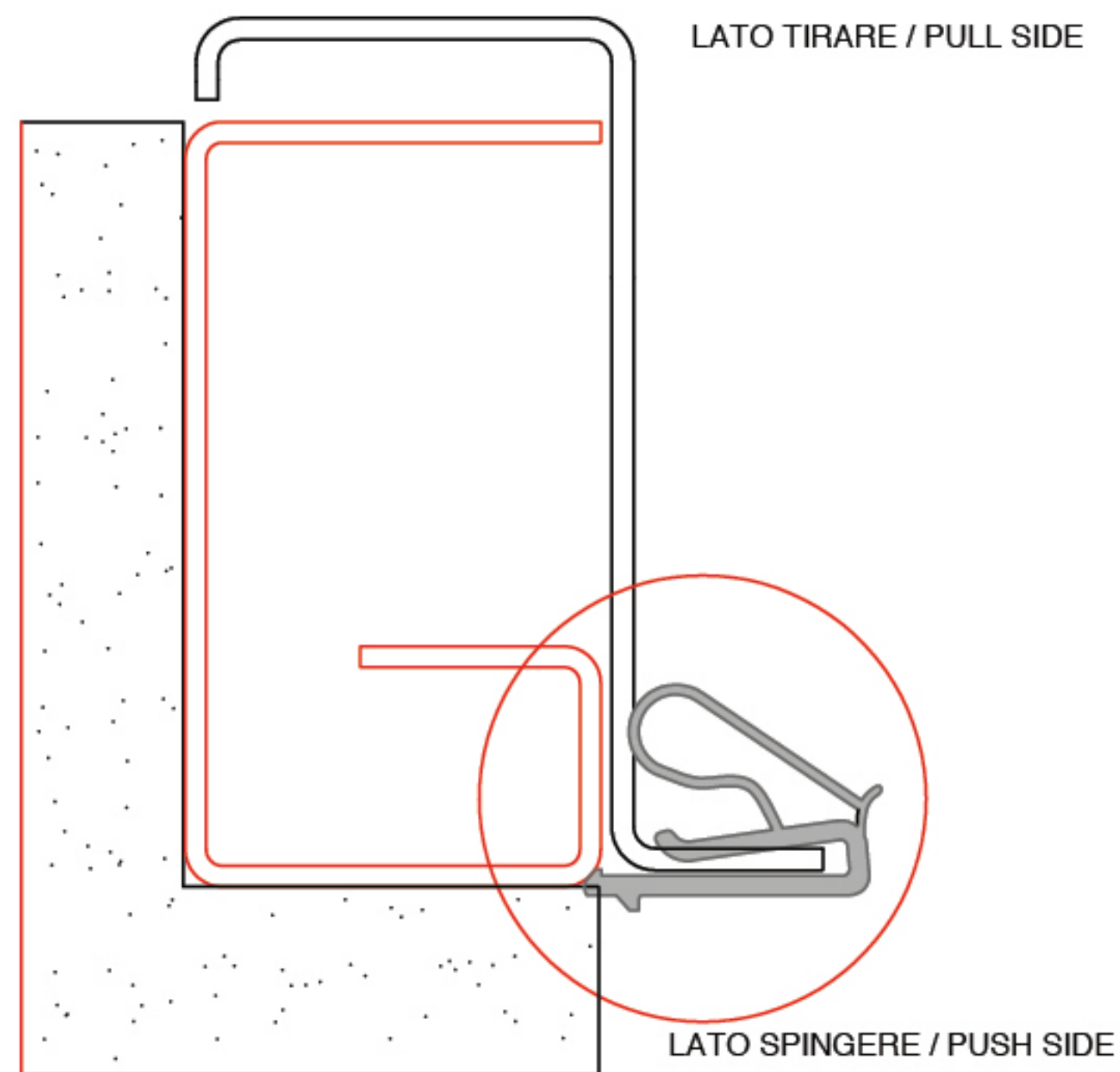
POSIZIONE GUARNIZIONE - Gasket position
