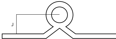
Maschietto fisso piego 17 mm Iron fixed double hinge fold 17 mm
