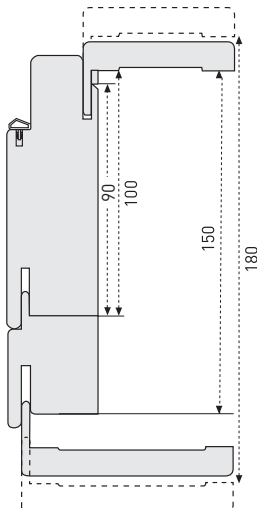
Telaio con ringrosso fino a 180 mm Frame with reinforcement up to 180mm
