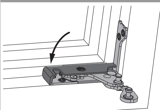
1. Aprire completamente il supporto cerniera
