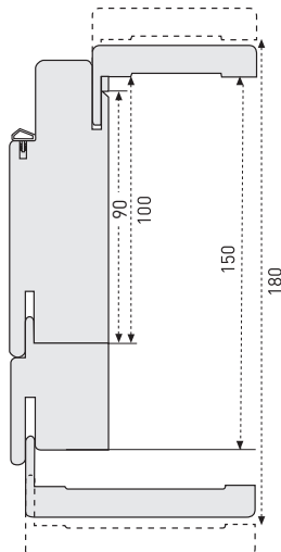
Telaio con ringrosso fino a 180 mm Frame with reinforcement up to 180mm
