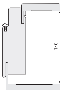
Telaio con coprifilo aletta lunga fino a 140 mm Frame with long-wing architrave up to 140mm
