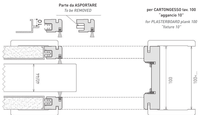
Particolare assemblaggio TRAVERSA CROSSPIECE assembly detail
