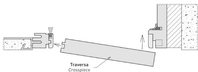
Particolare assemblaggio TRAVERSA CROSSPIECE assembly detail
