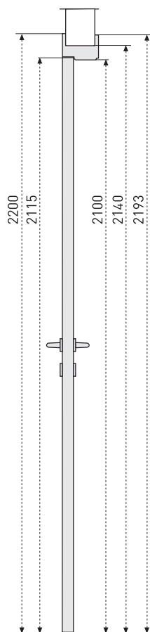
Telaio con ringrosso fino a 180 mm Frame with reinforcement up to 180mm
