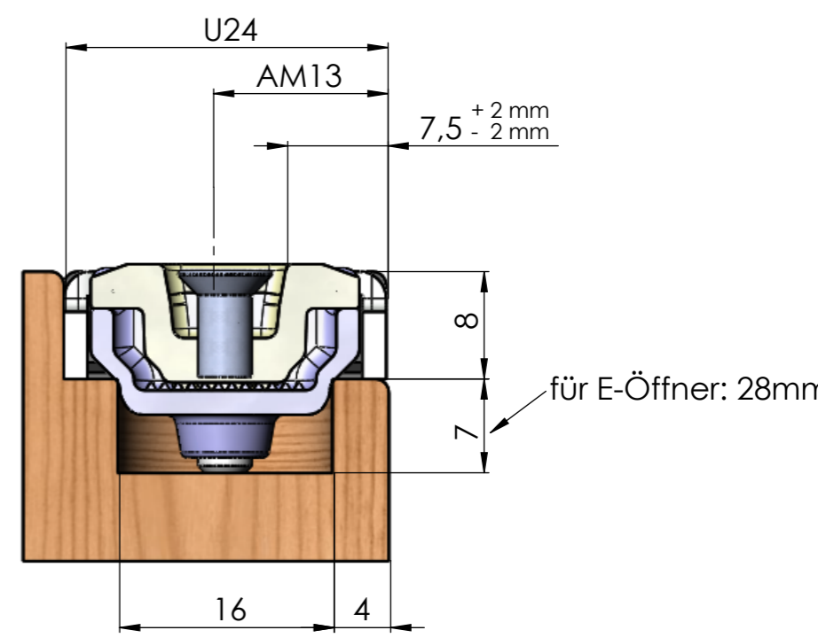
Einbaubeispiel M 2:1
